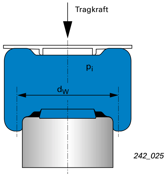
Schlauchrollbalg
