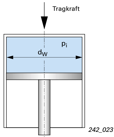
Schlauchrollbalg
