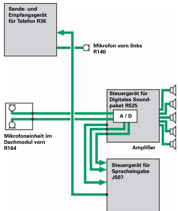
Mikrofonanordnung bei der Variante MMI-High
