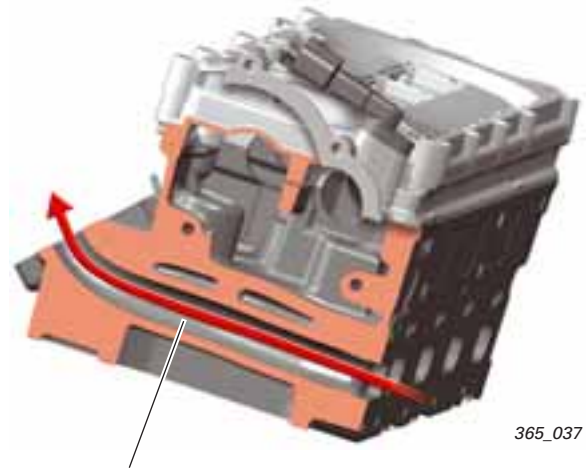
Abgaskanal vom Abgaskrümmern Vierzylinder durch den Zylinderkopf zum Abgasrückführungsventil
