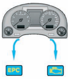
Блок управления комбинации приборов J285 с контрольной лампой электропривода акселератора K132 и лампой check engine K83
