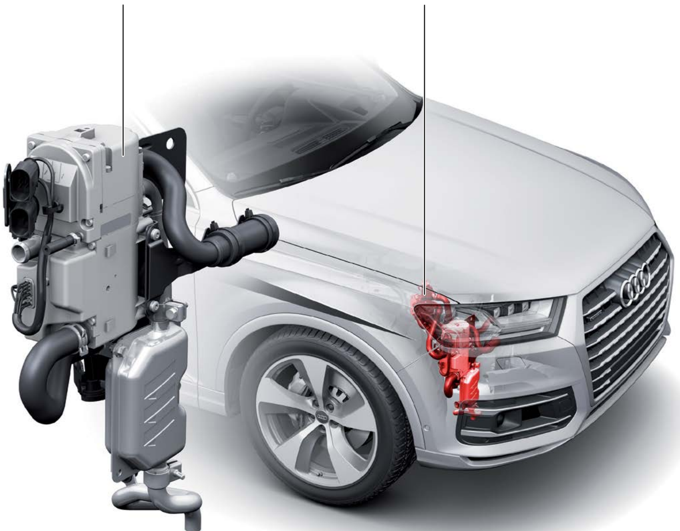
Нагревательный элемент дополнительного воздушного отопителя Z35 с блоком управления дополнительного воздушного отопителя J604
