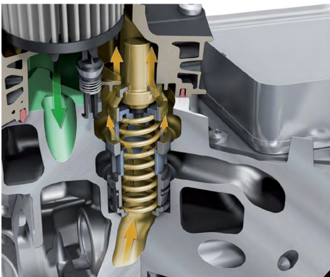
Перепускной канал закрыт: масло поступает к масляному фильтру напрямую в обход масляного радиатора
