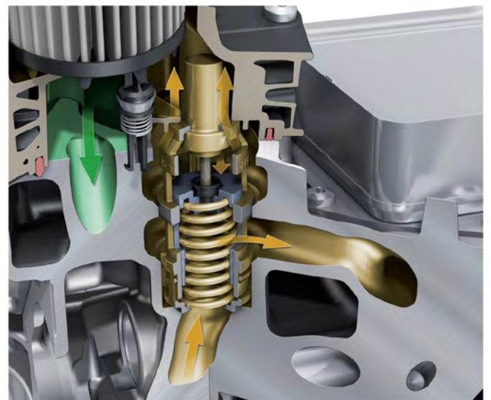
Перепускной канал открыт: масло проходит через масляный радиатор
