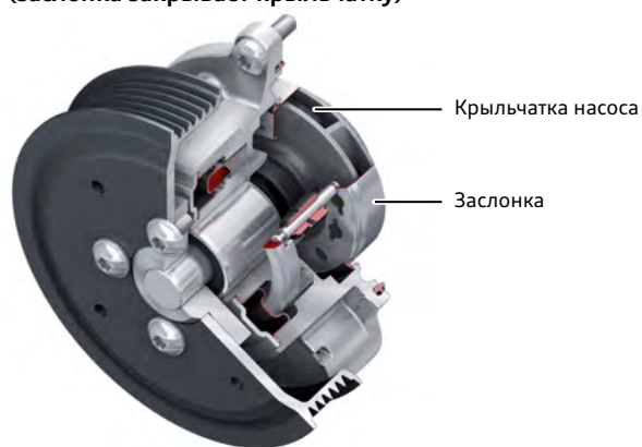
Насос охлаждающей жидкости закрыт (заслонка закрывает крыльчатку)
